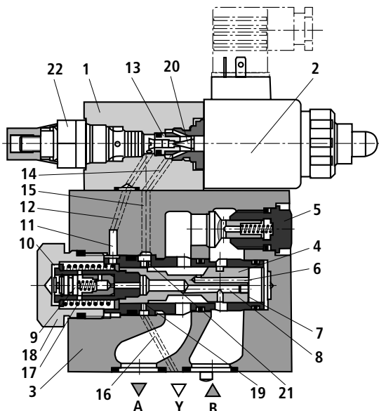
形式 DREM...-6X/...YG24K4... (チェック弁付き)
