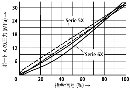
シリーズ 5X と 6X の比較 / 圧力設定範囲 31.5 MPa (800 mA コイル、アンプ VT-VSPA1-1-1X を使用)
