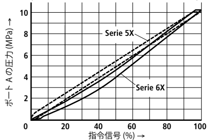
シリーズ 5X と 6X の比較 / 圧力設定範囲 10 MPa (800 mA コイル、アンプ VT-VSPA1-1-1X を使用)
