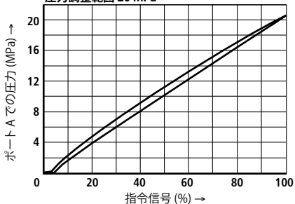
圧力調整方式 20 MPa (VT-SSPA1 使用)
