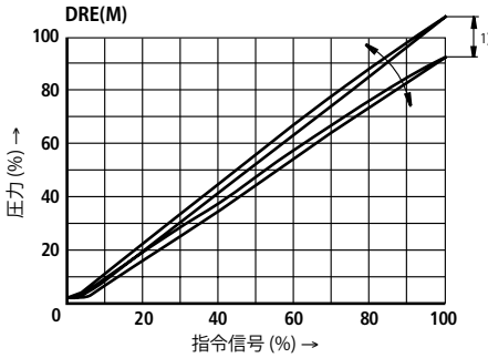
指令信号-圧力線図 (流量 = 0.8 l/min)
