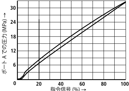
圧力調整範囲 31.5 MPa
